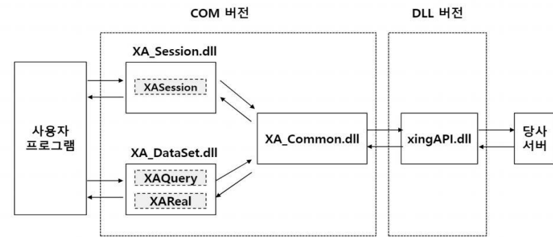
※ COM 구성도
